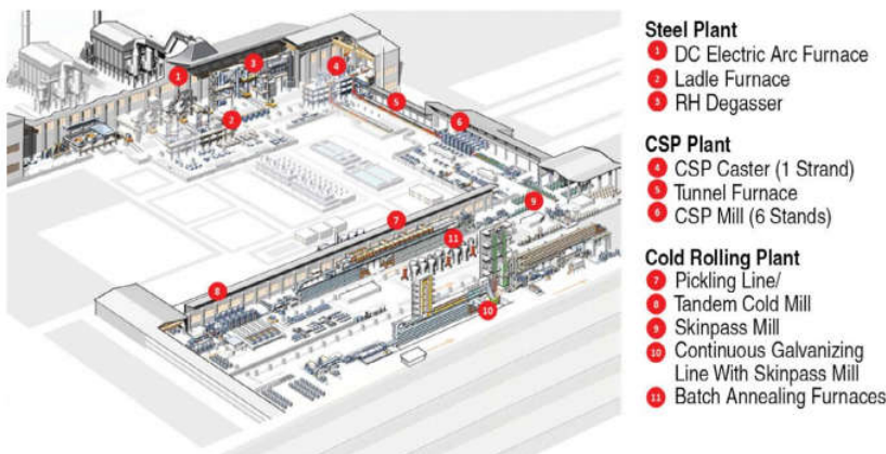
شکل 1- نمای کلی مجتمع مینی میل BRS.
