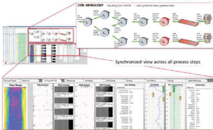
شکل 3 - PQA - مانیتور کیفیت محصول که زنجیره کامل فرآیند را پوشش می‌دهد (از فولادسازی تا فرآوری نهایی).
